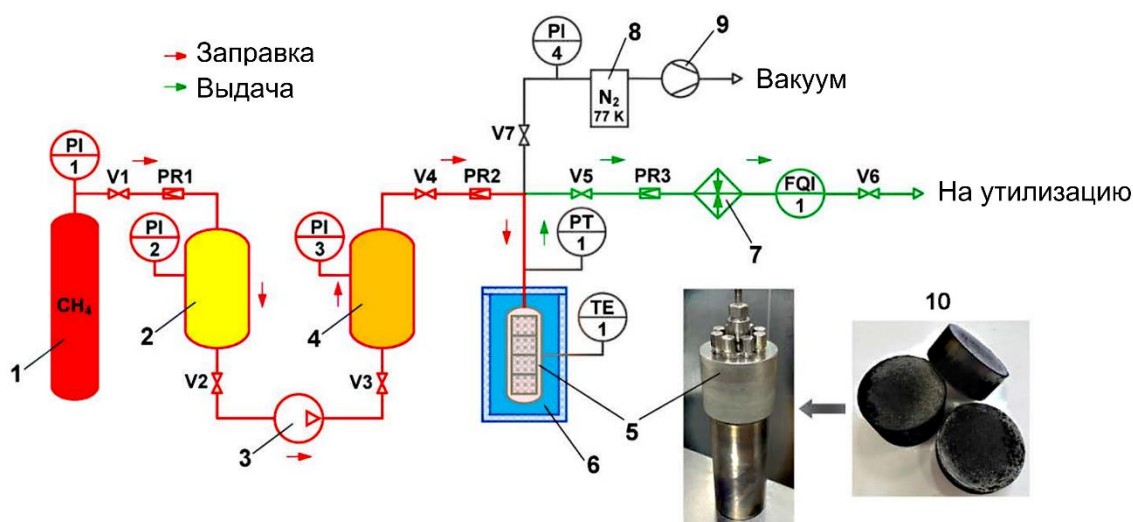
Рисунок 2.3. Принципиальная схема экспериментального стенда для измерения удельных объемных характеристик адсорбционного аккумулятора.
