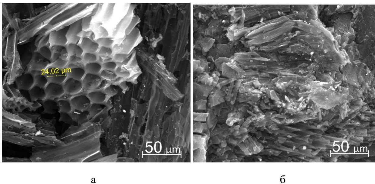
Рисунок 3.8. Микрофотографии образцов S-1М (а) и S-1М-КМЦ-ГК (б).
