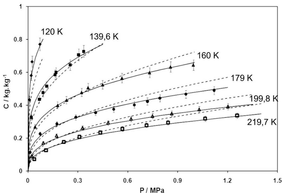
Рисунок 1.6. Изотермы адсорбции метана при температурах 120-220 К на адсорбенте MAXSORB-III [92].
