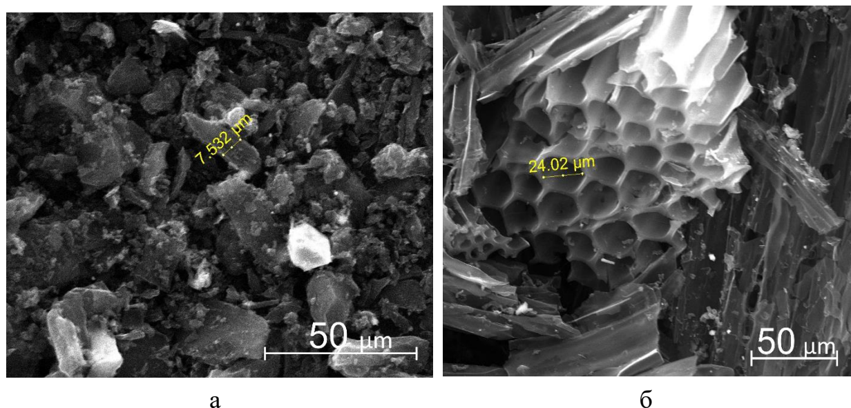
Рисунок 3.2. Микрофотографии образцов ES-1М (а) и S-1М (б).
