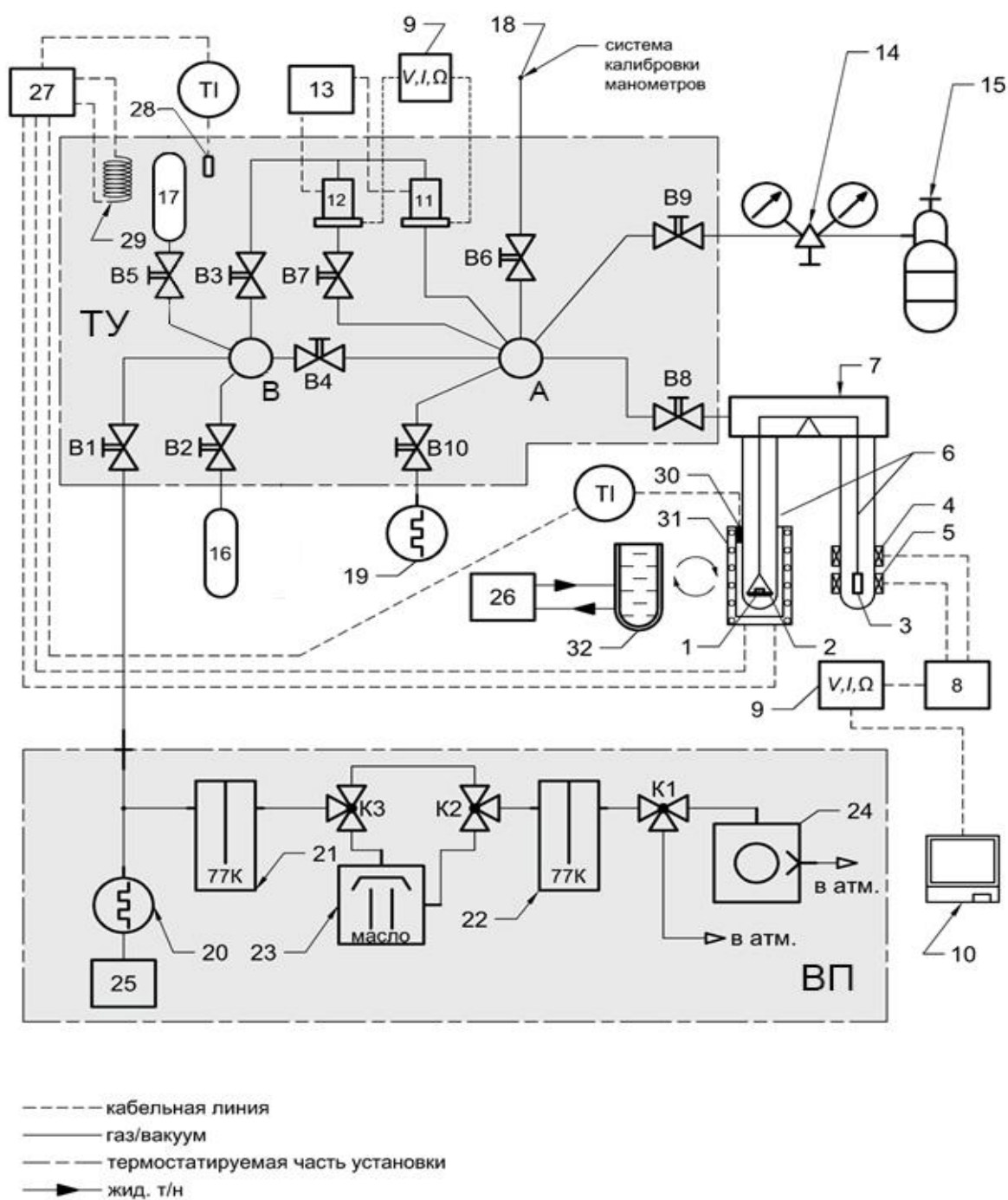
Рисунок 2.2. Принципиальная схема стенда СТ-5.001-АГМ
