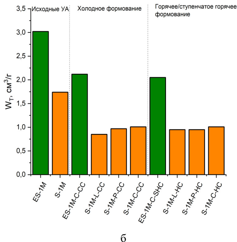
Рисунок 3.10. Зависимость плотности (а) и суммарного объема пор (б) полученных адсорбентов от параметров компактирования. Зеленый цвет – серия образцов ES-1M; Оранжевый цвет – серия образцов S-1M.
