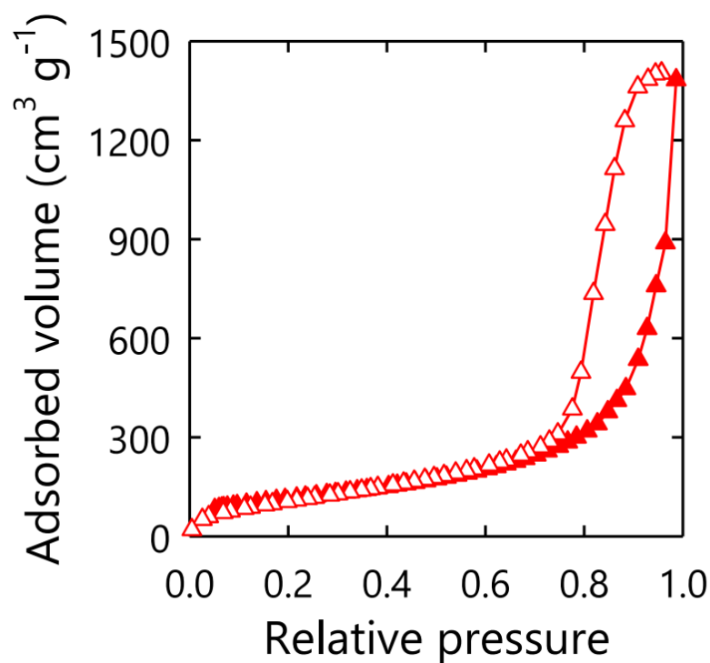
Рисунок 1.4. Изотерма адсорбции азота на углеродном ксерогеле полученном из целлюлозных нановолокон [86].
